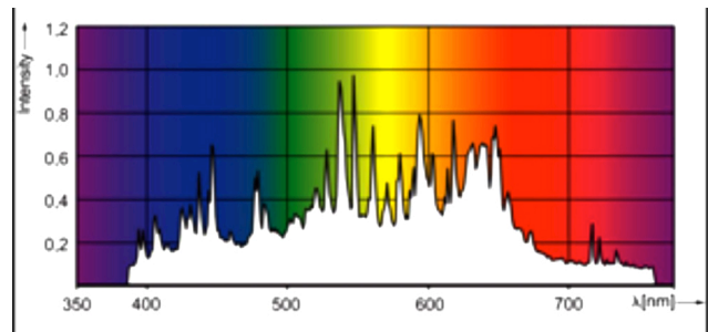
4200k - 315W Lamp (BUcMh31542K)
